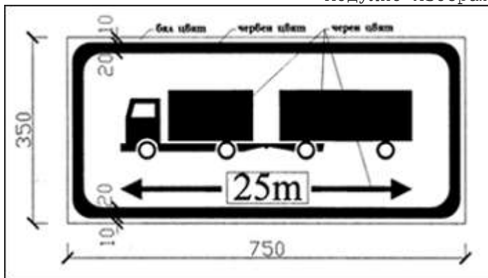
Табела за обозначаване действителната дължина на пътно превозно средство в m (на табелата е означена примерна дължина)
