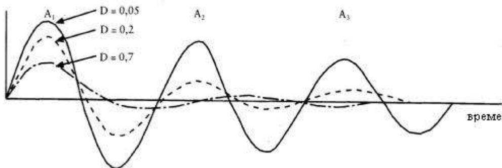
Фиг. 1. Синусоидална крива при свободни и краткотрайни трептения Честотата може да бъде изчислена чрез измерване на времето до момента,
